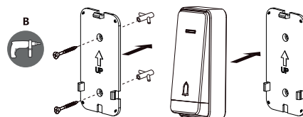
Ruuvikiinnitys
