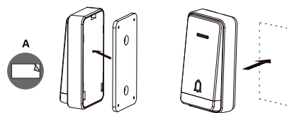
Teippikiinnitys
