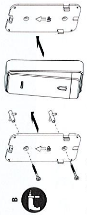
Ruuvikiinnitys
